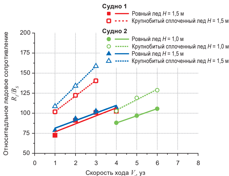
Рис. 5. Сопоставление данных измерений ледового сопротивления крупнотоннажных судов класса Arc7 при движении в ровном (сплошные линии) и сплоченном крупнобитом льду (пунктирные линии)
