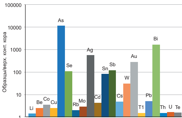
Рис. 3. Распределение основных микроэлементов (среднее по изученным образцам рудопроявления Палянгай), данные ИСП МС, нормированные по отношению к средним значениям для верхней коры [9]
