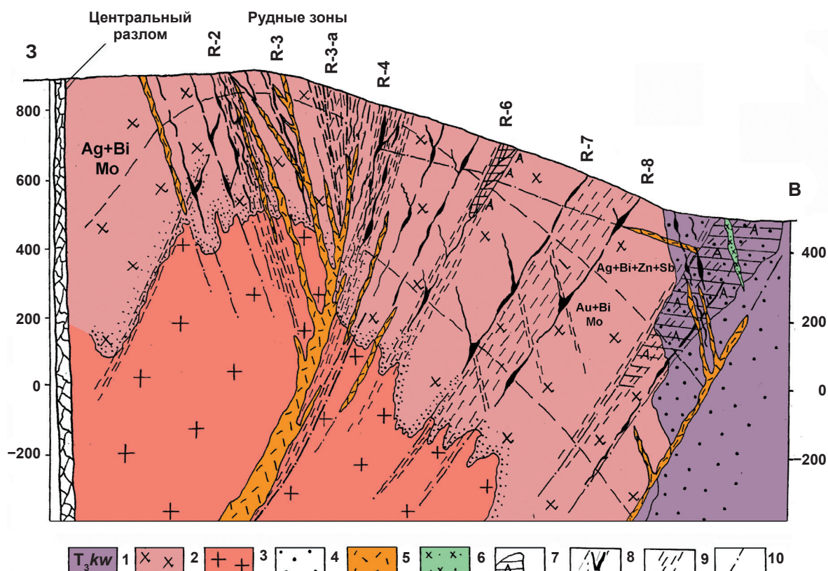
Рис. 2. Схематический геологический разрез в крест простирания рудных зон рудного поля Палянгай (по [4] с изменениями и дополнениями): 1 – алевриты и песчаники верхнего триаса, 2 – гранодиориты, 3 – граниты, 4 – роговики, 5 – дайки риолитов, 6 – дайки диоритов, 7 – аргилитовые метасоматиты, 8 – рудные зоны, 9 – зоны трещиноватости, 10 – разломы Fig. 2. Schematic geological cross-section of the strike of ore zones of the Palyangai ore field (after [4], with modifications and additions): 1 – siltstones and sandstones of the Upper Triassic, 2 – granodiorites, 3 – granites, 4 – hornfelses, 5 – rhyolite dikes, 6 – diorite dikes, 7 – argylized metasomatites, 8 – ore zones, 9 – fracturing zones, 10 – faults
