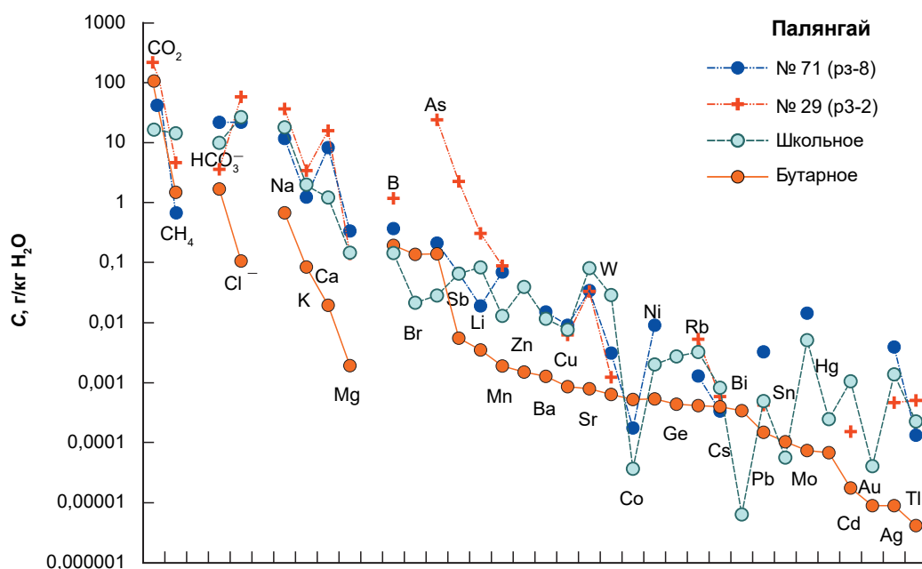
Рис. 5. Сравнение химического состава рудообразующего флюида рудопроявления Палянгай (пробы № 71 и 29) с составом флюида месторождений Школьное и Бутарное (см. табл. 3)
