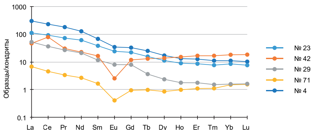
Рис. 4. Распределение REE, нормированных по хондритам [10], в изученных образцах рудопоявления Палянгай. Характеристика проб приведена в примечании к табл. 1
