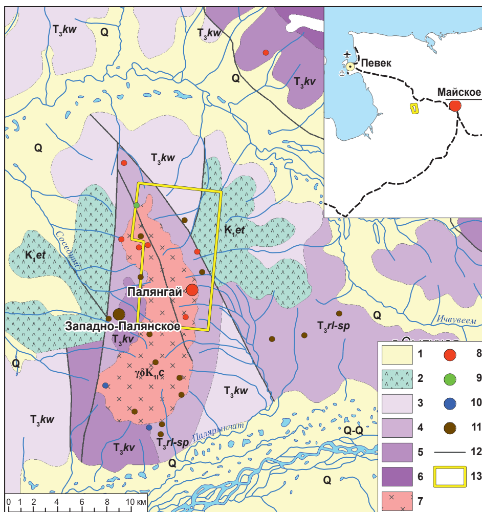
Рис. 1. Геологическое строение Палыангайской площади: 1 — четвертичные аллювиальные отложения; 2 — вулканогенные комплексы среднего и основного состава этчикунской свиты нижнего мела; 3–5 — верхний триас: 3 — песчаники и алевролиты кувеемской свиты, 4 — песчаники, алевролиты и реже сланцы релькувеемской свиты, 5 — песчаники и алевролиты кувеемской свиты; 6 — алевролиты, глинистые сланцы, кварц-полевошпатовые песчаники ичувеемской свиты нижнего триаса; 7 — гранодиориты чукотского комплекса раннего мела; 8–11 — месторождения и проявления: 8 — золоторудные и золото-серебряные, 9 — медные, 10 — полиметаллические, 11 — цветные (ртутные, оловорудные, вольфрамовые, висмутовые); 12 — разрывные нарушения; 13 — границы лицензионной площади
